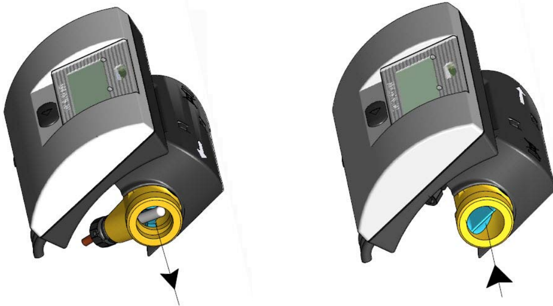
Рис. 5: Монтаж счетчика с резьбовым присоединением
