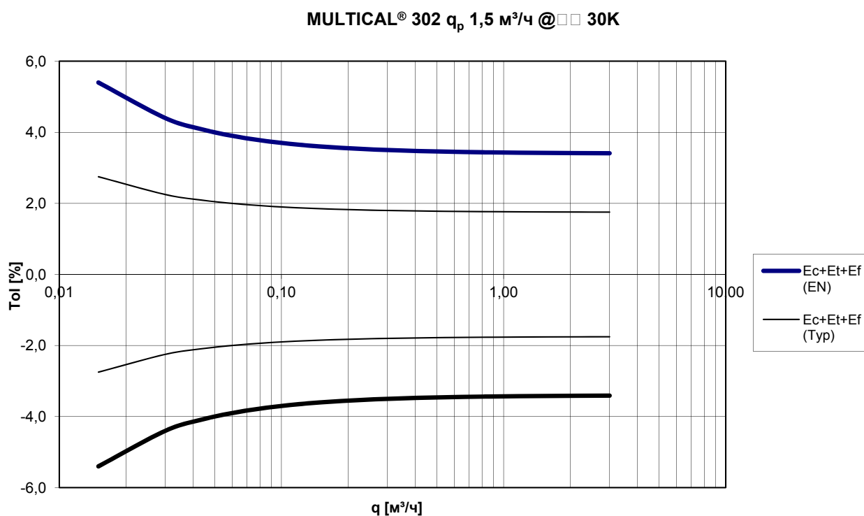
Схема 1: Общая точность измерений MULTICAL® 302 s® в сравнении с требованиями EN 1434-1.
